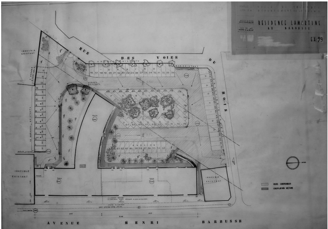
Plan masse. Fonds Lesné-Bernadac.
