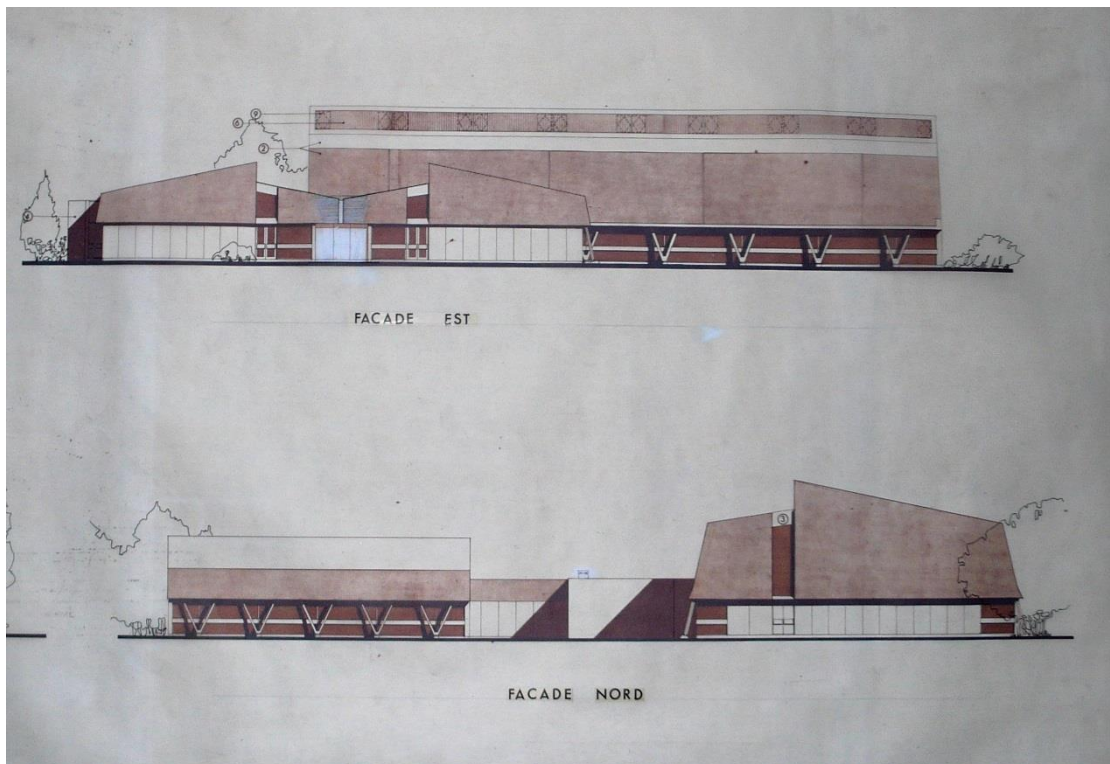
Façades est et nord, calques. Fonds Lesné-Bernadac.
