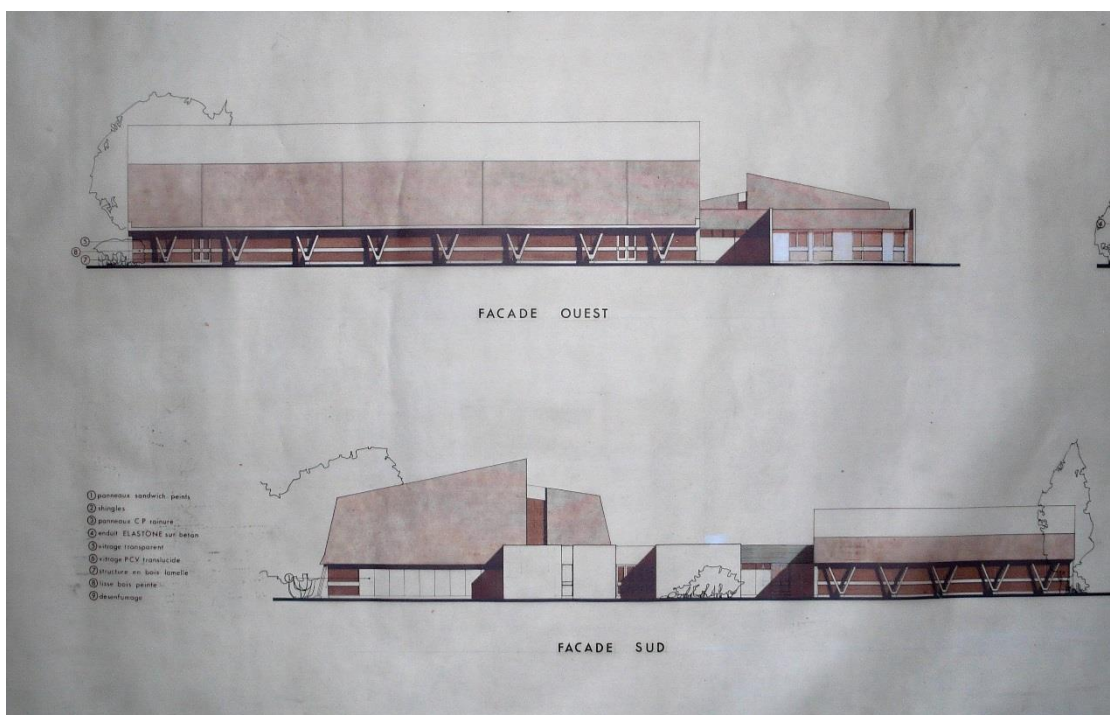
Façades ouest et sud, calques. Fonds Lesné-Bernadac.
